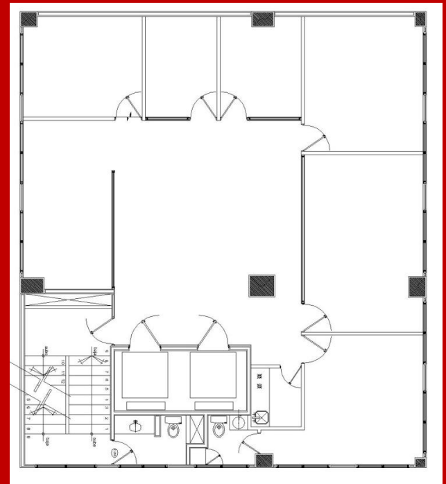
PLANTA TIPO
